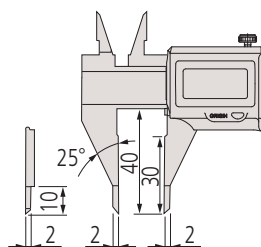
Vékony mérőcsőrrel
