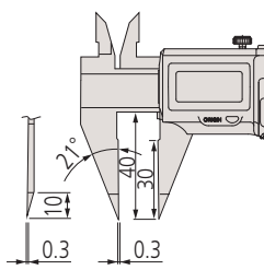
Hegyes mérőcsőrrel
