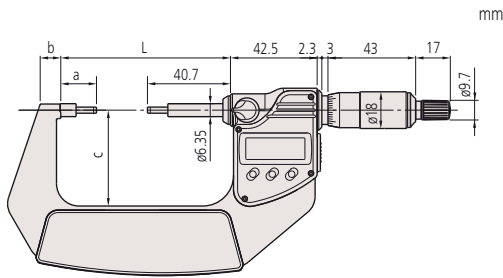
0-75 mm
