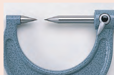
Csúcsszög: 30°
