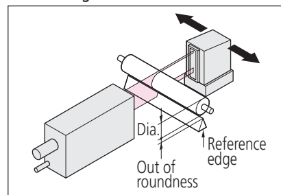
Henger külső átmérőjének és kőrkőrősségének mérése
